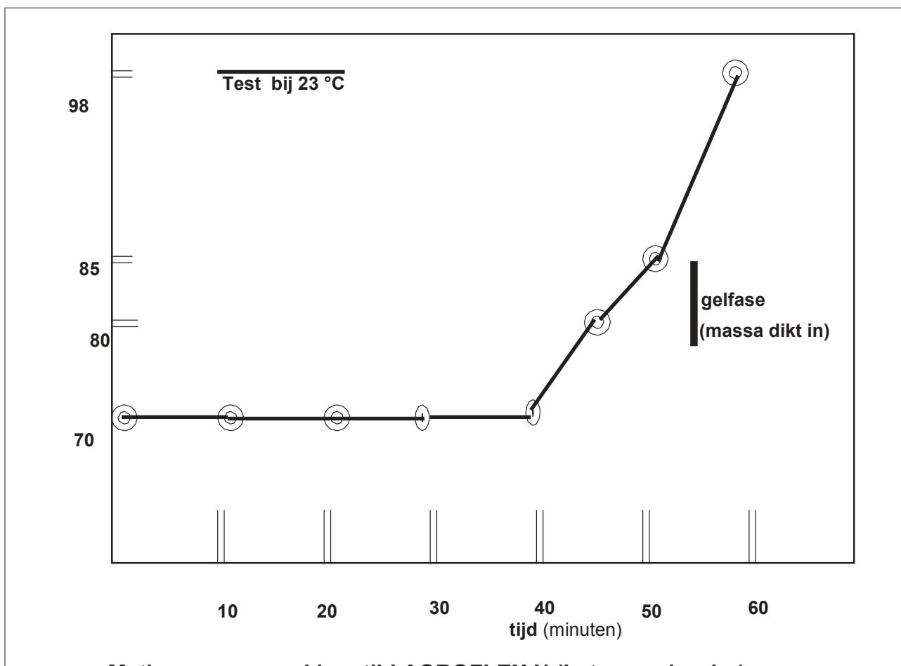
Meting van verwerkingstijd AGROFLEX N (Latex+verharder)
